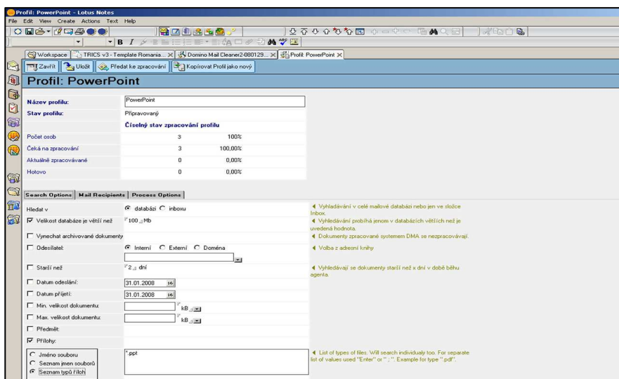
Obr. 2 – Vyhledávací podmínky
