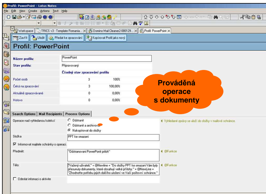
Obr. 1 – Nastavení procesu
